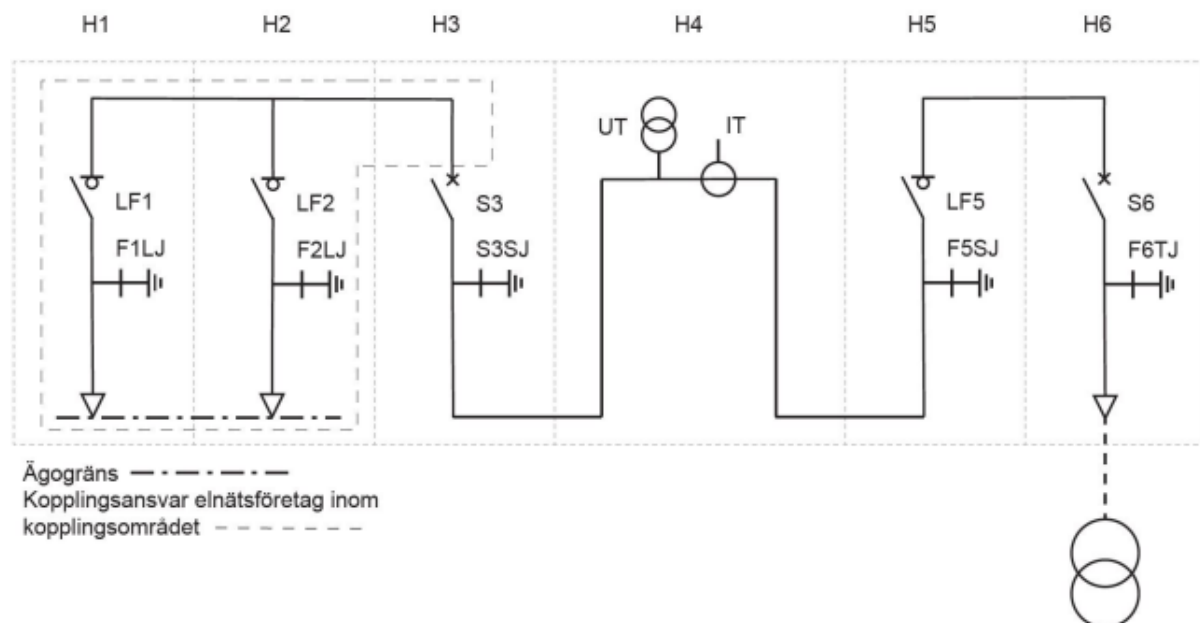
Bild 1. Principskiss för enlinjeschema
